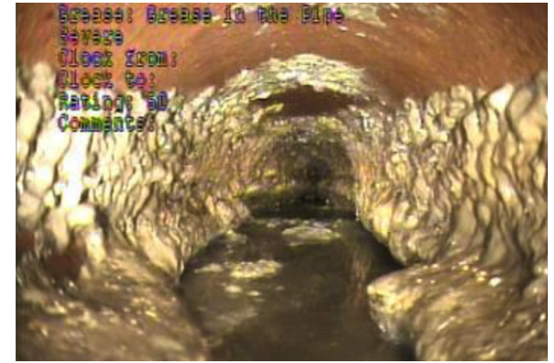
Esta foto del interior de una tubería de alcantarillado en Walla Walla muestra cómo se acumula la grasa, aceite y manteca.
